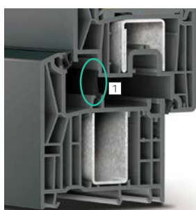
1 uszczelka środkowa
